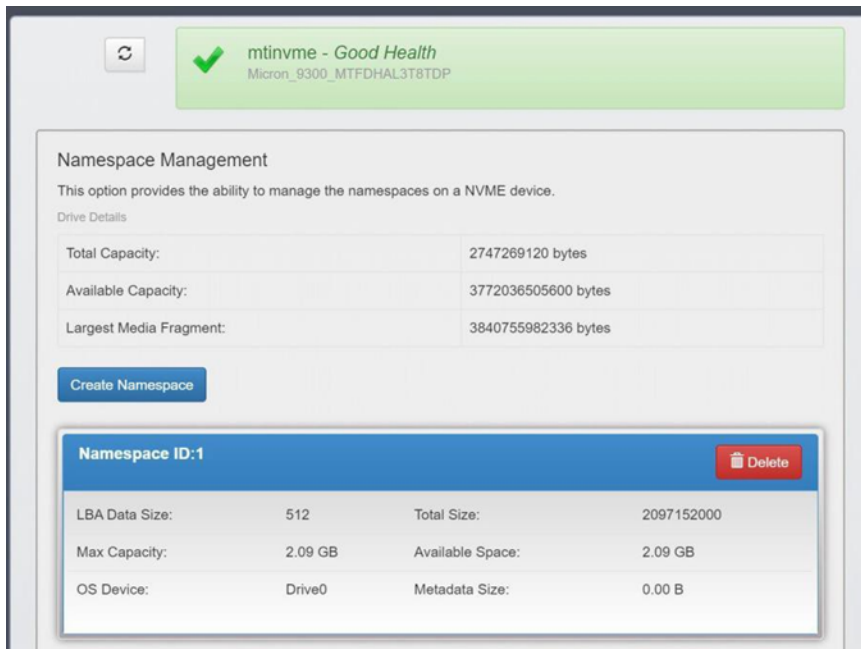
Fig: 26 Namespace Management
