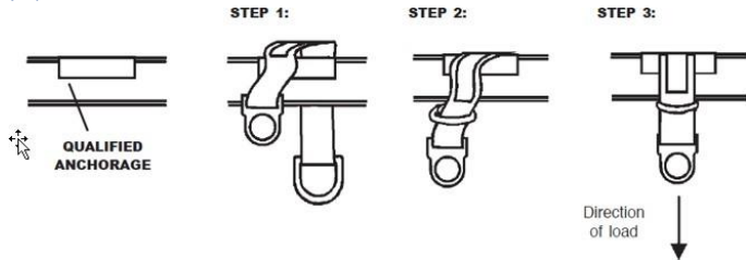
图8 多次包裹锚固点 以缩短长度。每包裹一层均将小D型环穿过大D型环。
