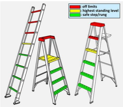
图26 用梯规范
